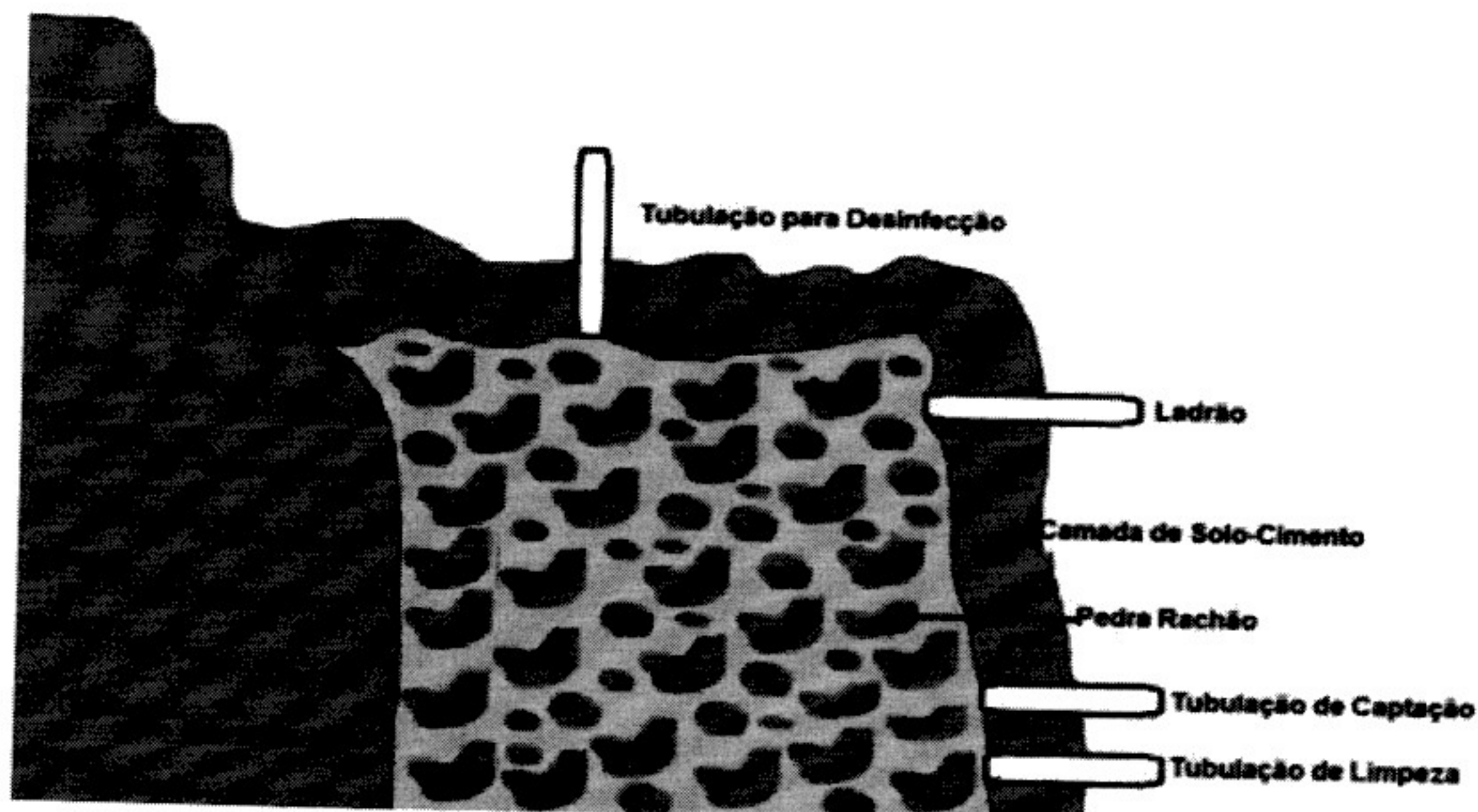
Figura 8 - Esquema ilustrativo recuperação de nascentes
