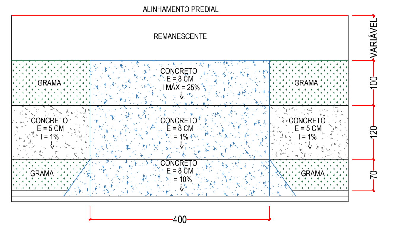
DETALHE ACESSO DE VEÍCULOS ESCALA 1 : 50
