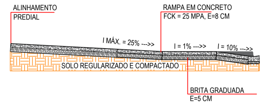
CORTE ACESSO DE VEÍCULOS ESCALA 1 : 50
