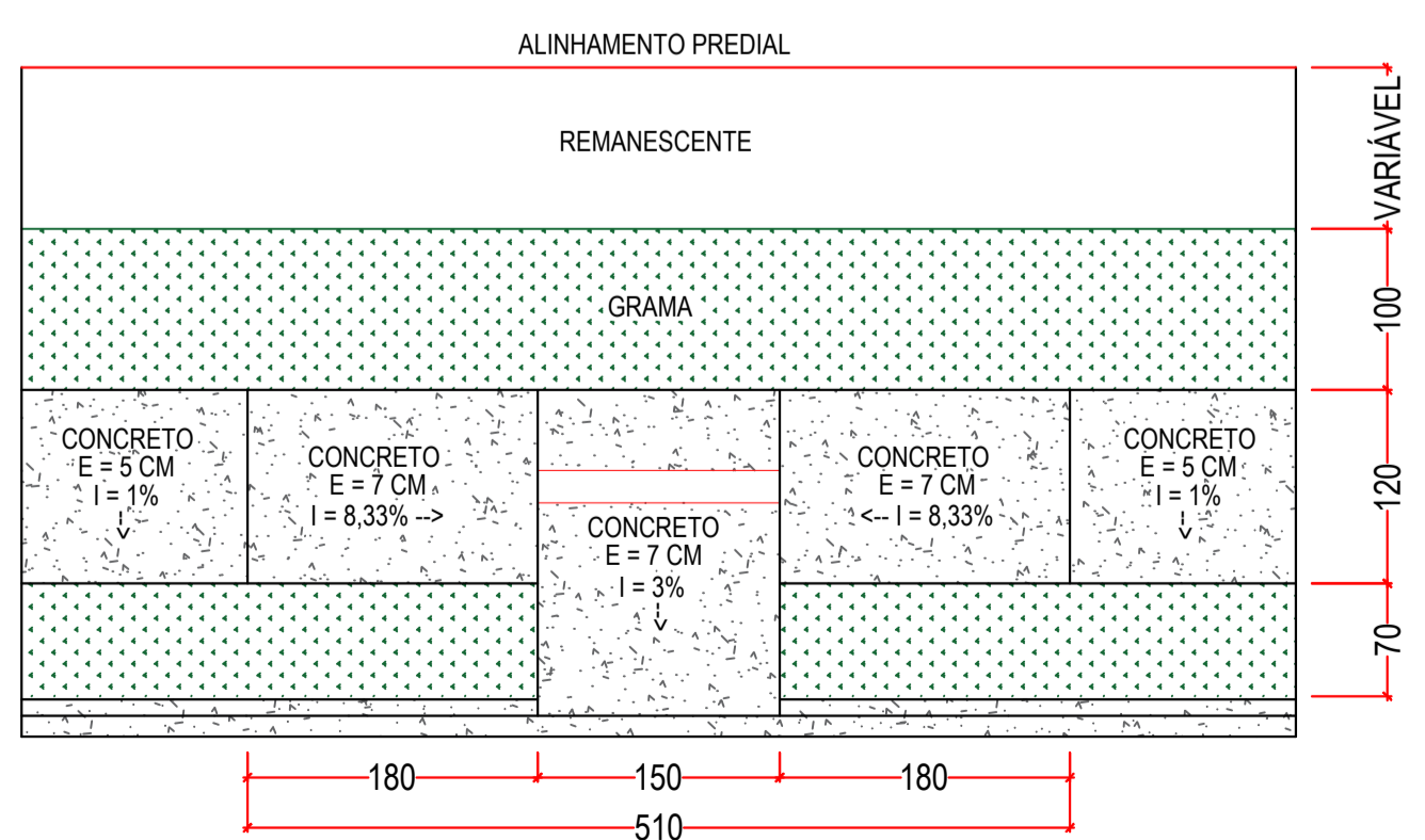
DETALHE RAMPA DE ACESSIBILIDADE ESCALA 1 : 50
