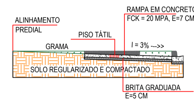
CORTE RAMPA DE ACESSIBILIDADE ESCALA 1 : 50
